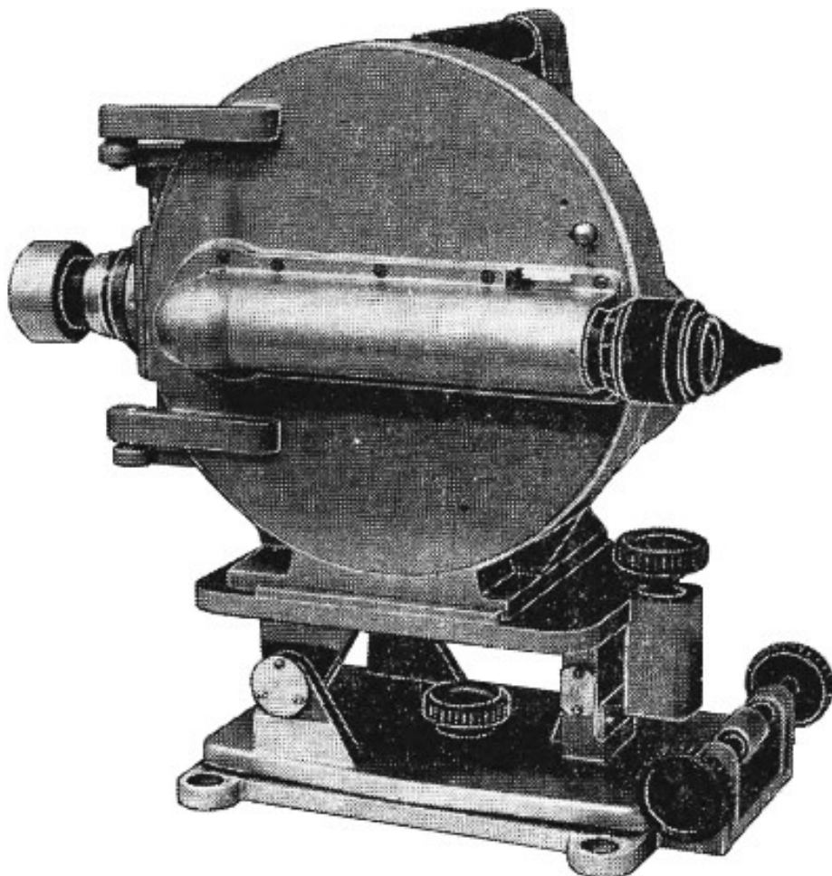
Рис. 7. Камера СКС-1М на подставке
