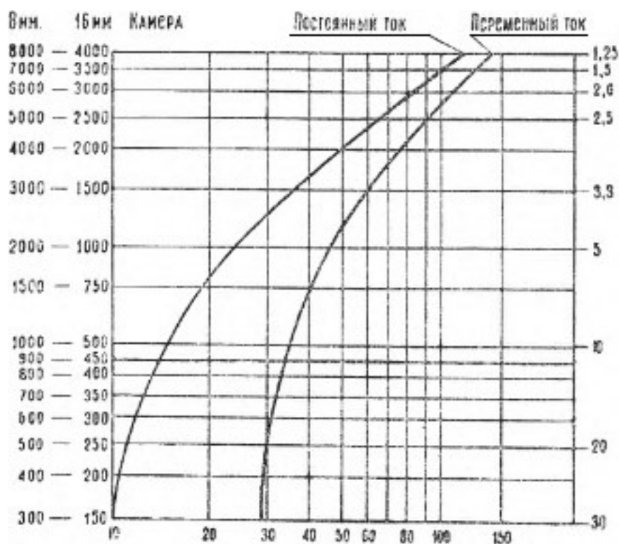
Рис. 9. Типовая диаграмма зависимости скорости и времени от напряжения Диаграмма дает ориентировочную зависимость скорости от напряжения. При необходимости иметь точную зависимость, нужно составить диаграмму специально для каждой камеры.
