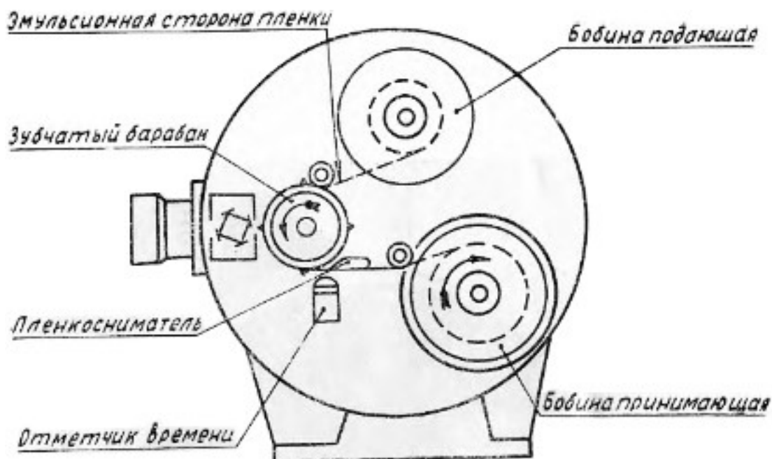
Рис. 1. Схема зарядки киноплёнки
