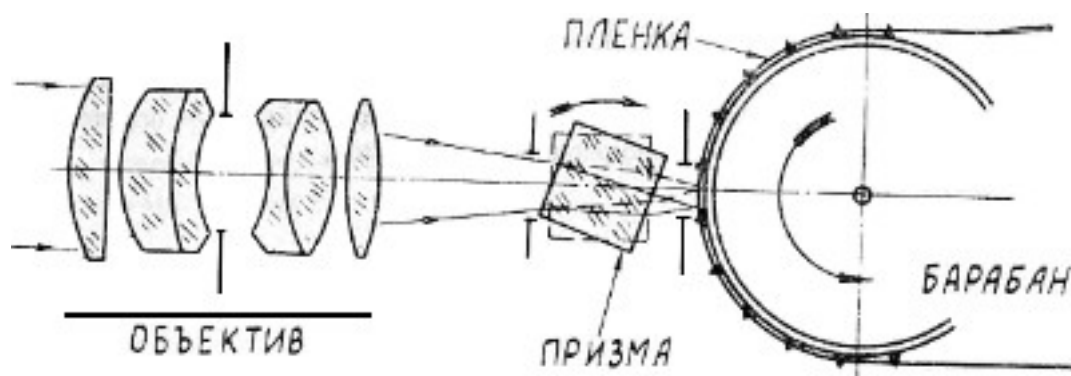
Рис. 2. Схема оптики
