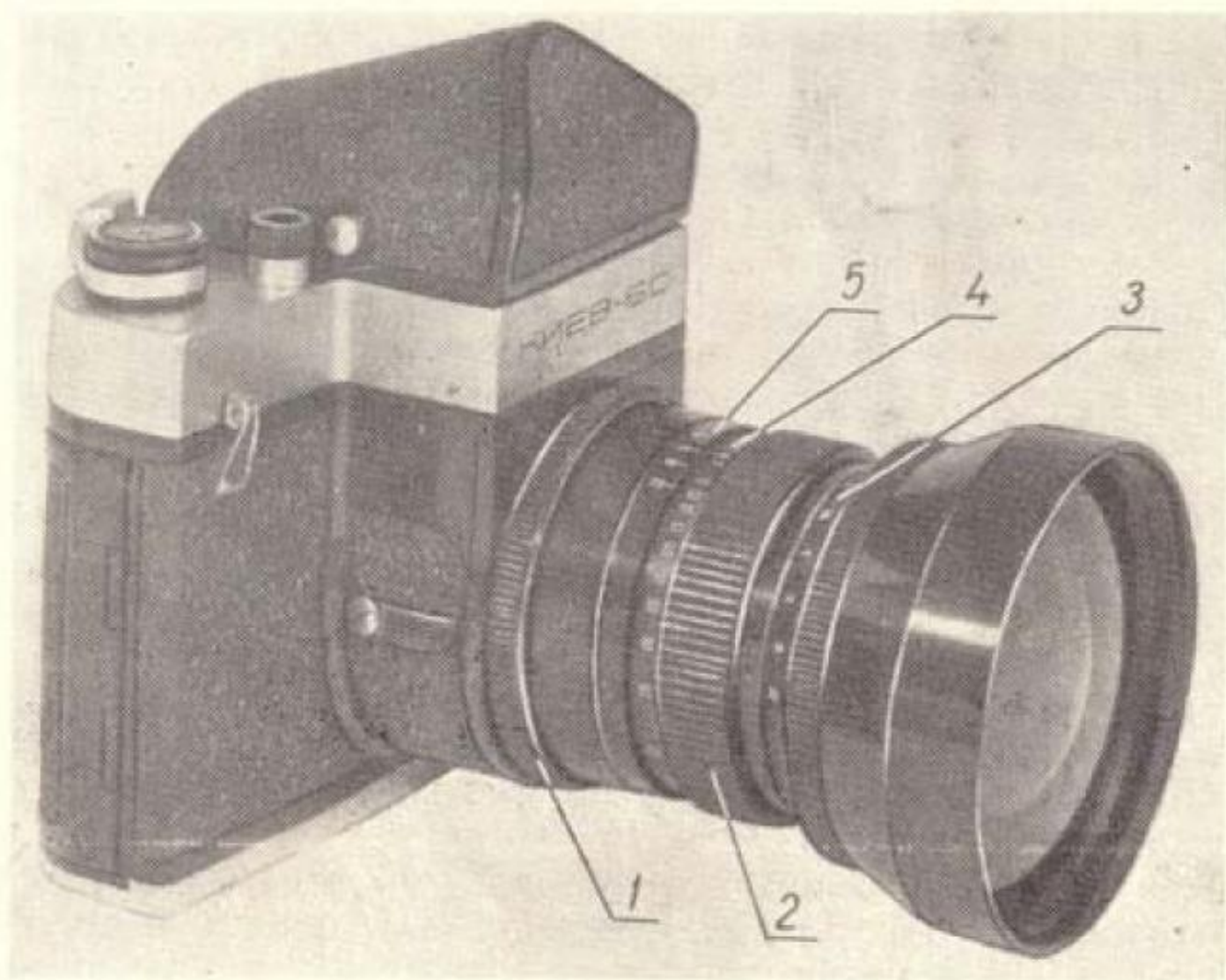
Рис. 1. Фотоаппарат «Киев-6С» с объективом «Мир-3Б»
