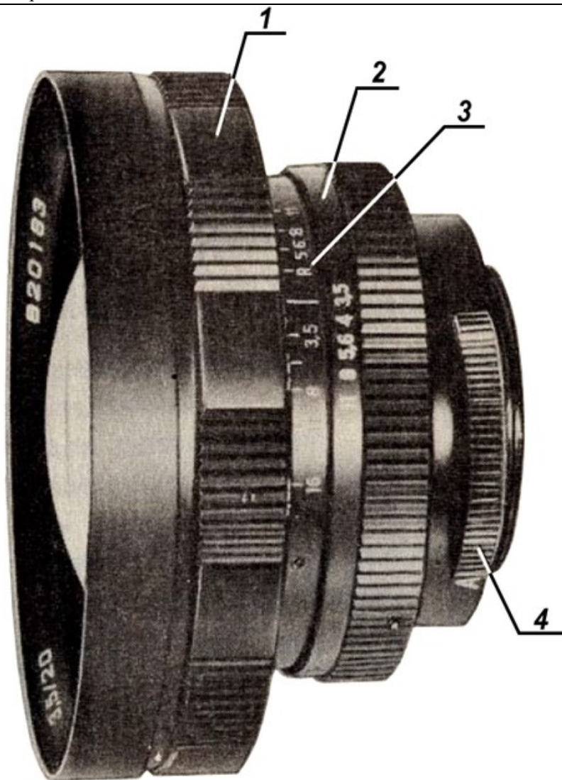
Рис. 2. Общий вид объектива
