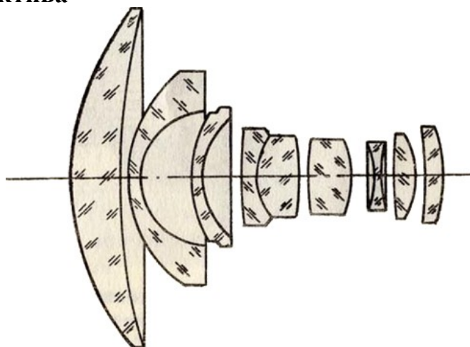
Рис. 1. Оптическая схема объектива
