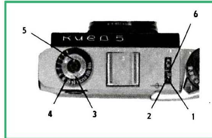
Рис. 20. Будова експонетра:
