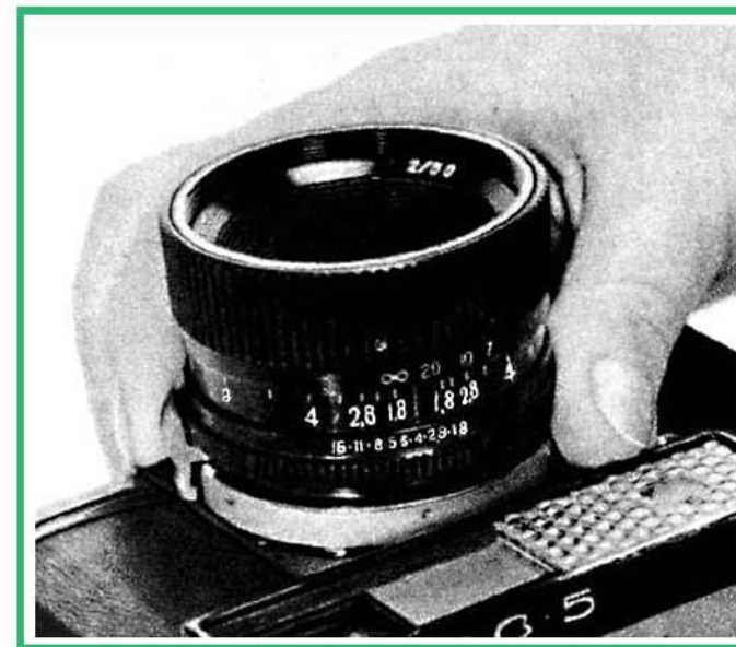
Рис. 21. Знімання об'єктива.
