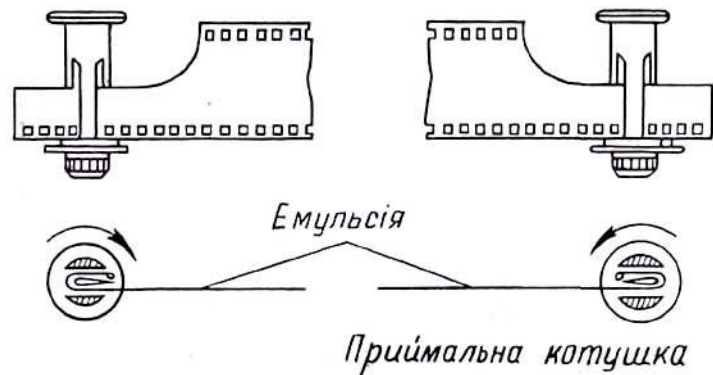
Рис. 7. Схема заправки плівки.
