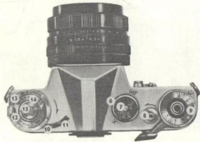
6—диск синхронизации; 7—диск выдержек затвора; 8—втулка отключения затвора; 9—лимб счетчика кадров; 10—стрелка измерителя экспонометра; 11—стрелка калькулятора; 12—шкала светочувствительности пленки; 13—шкала выдержек калькулятора; 14—шкала диафрагм калькулятора; 15—головка обратной перемотки
