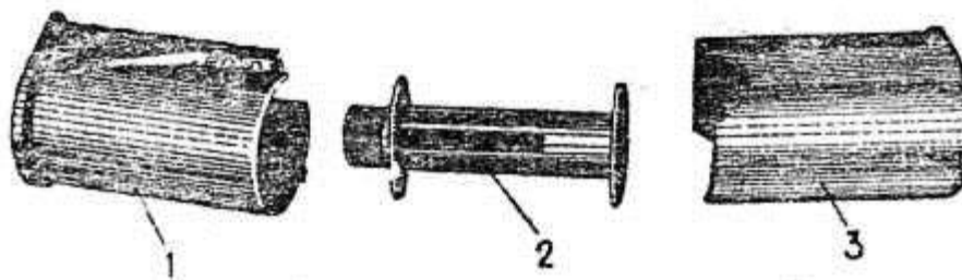
Рис. 4. Кассета фотоаппарата «Кристалл»: 1 – гильза, 2 – катушка, 3 – обойма (корпус кассеты).
