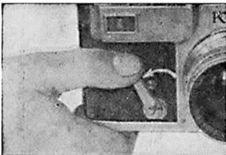
Рис. 25. Взвод рычага самоспуска.
