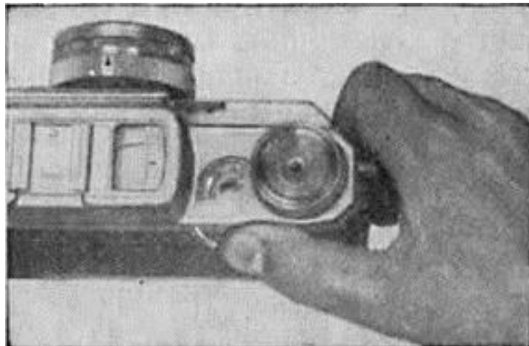
Рис. 15. Установка счетчика на „0“.
