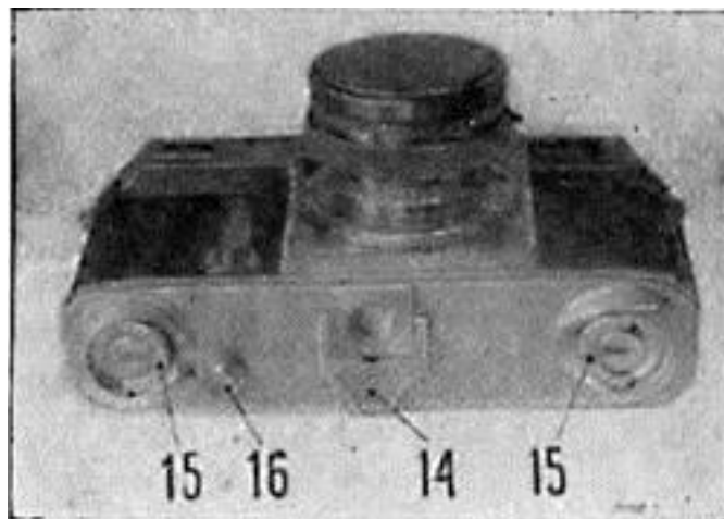
Рис. 2. Вид аппарата снизу.
