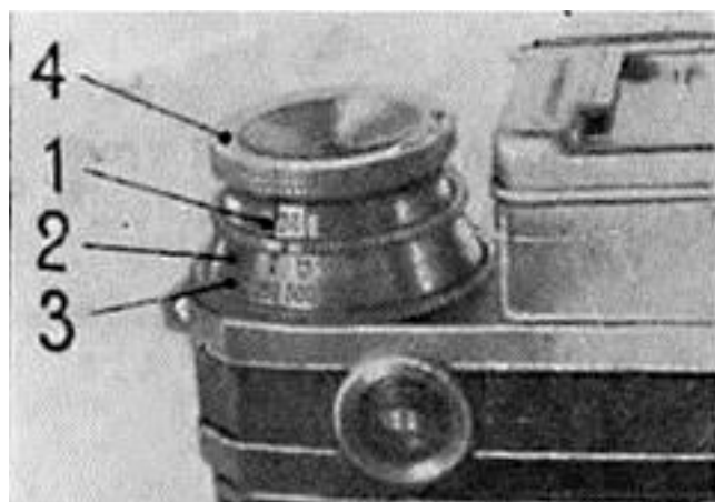
Рис. 34. Головка обратной перемотки мод. III.
