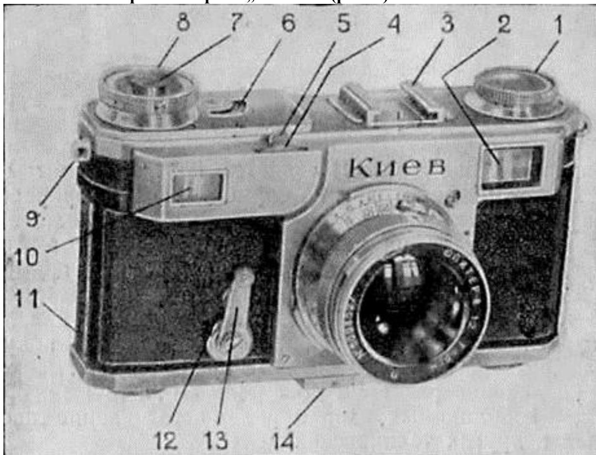
Рис. 1. Общий вид фотоаппарата „Киев“-II
