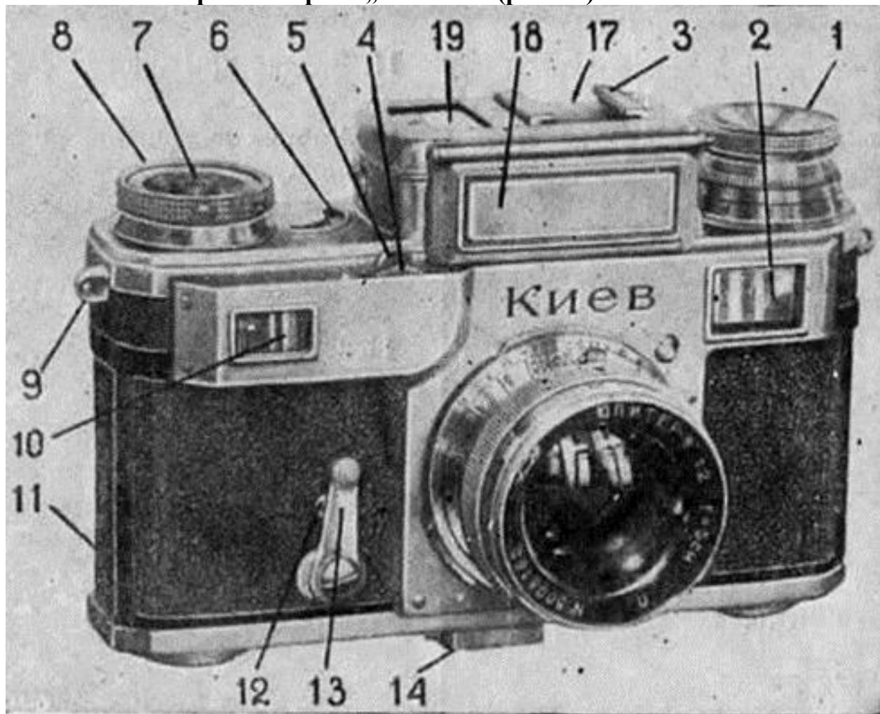
Рис. 31. Общий вид фотоаппарата „Киев“-III.
